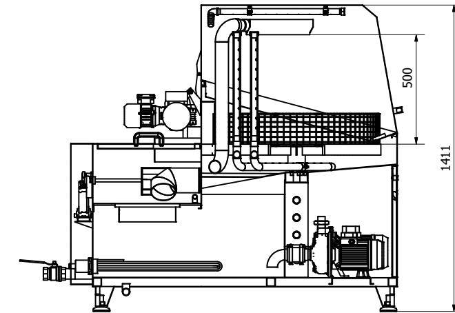
L-L ( 1 : 12 )
