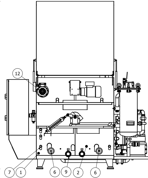
L-L ( 1 : 12 )
