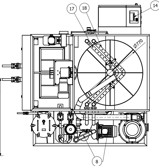
A-A ( 1 : 11 )
